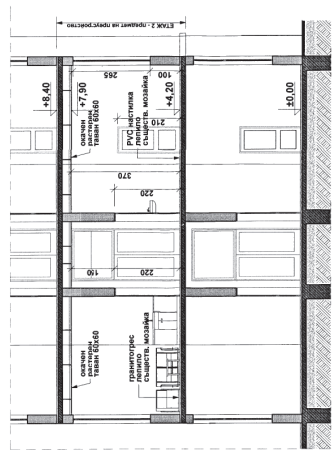
ВЕРТИКАЛЕН РАЗРЕЗ 1-1
